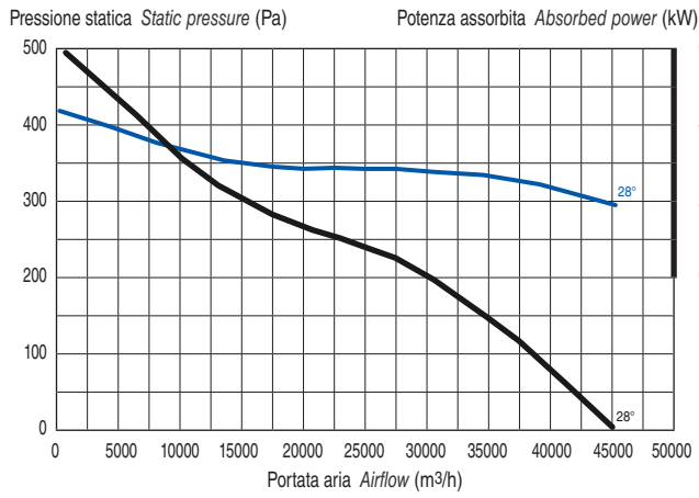
mod. 1126/B · 4 kW Potenza installata Motor power
