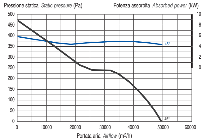
mod. 1006/C · 5,5 kW Potenza installata Motor power
