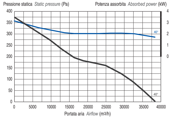
mod. 1006/B · 3 kW Potenza installata Motor power
